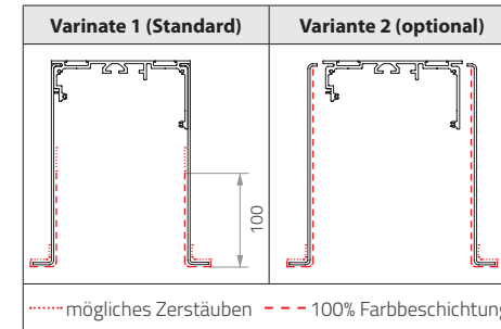
Kasten-Lackierung – Varianten
